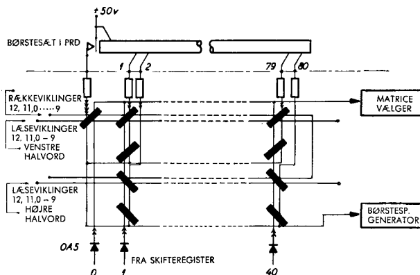
Fig. 5. Principskema for bufferregistre for aflæsning af kort. De ulige kolonner indlæses i øverste halvdel og de lige kolonner i nederste halvdel af matricen. De 24 læseviklinger er koblet i serie for alle 4 læsematricer. Rækkeviklingerne er i serie i alle 5 matricer. Pilene angiver strømretning og deres antal vindings-tallet
