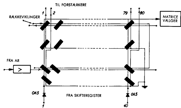
Fig. 10. Principskema for ferritkernematrix til styring af blokhulleren.
