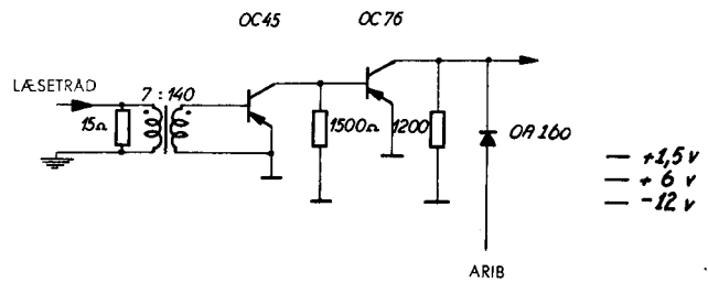
Fig. 9. Læseforstærker.
