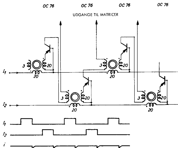
Fig. 8. Princip for skiftregister. Skiftregistret virker som en art omskifter, der for hver impuls går et trin frem og kobler den følgende strømimpuls til næste trin.
