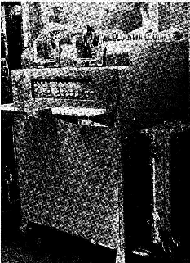
Fig. 2. Reproduktionsmaskine Bull-PRD. Man ser de to kortmagasiner foroven og ledningerne til børstesættene. Forneden til højre koblingstavlen, hvorover alle forbindelser er ført.
