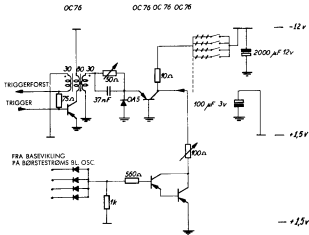
Fig. 7. Rækkestrømsgenerator. Den øverste blokeringsoscillator giver strøm til aflæsning af hullematricen i begyndelsen af hvert punkt, medens de nederste to transistorer giver rækkestrøm midt i punktet ved aflæsning af kort. Øverst til højre ses PRD's selecteur, som vælger række.
