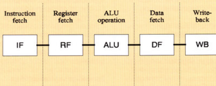
Figur 1. Pipelinen i en R3000-processor består af 5 trin. Det giver mulighed for at op til 5 instruktioner udføres samtidig. Hvert enkelt trin varer 30-40 ns.
