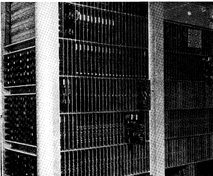
Fig. 8. GIER-centralenhedens praktiske opbygning. Pladerne med trykte kredsløb er anbragt i skuffer og forsynede med 30-polede stik. Yderst til venstre ses styreenheden med toroidkernerne og mikroprogramtrådene. Foroven i styreenheden, der er ophængt i et hængsel og kan svinges ud af skabet, ses en plade med dioder til afkodning af de valgte tråde.
