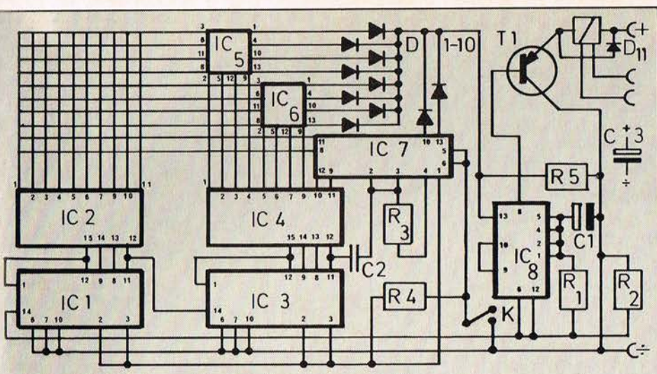
Diagram AUTOFON.
