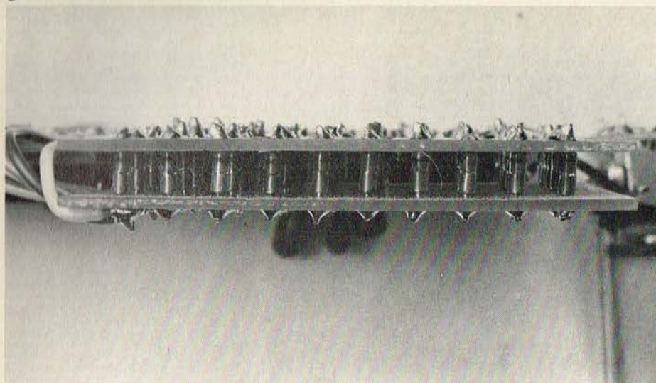
Diodematrix med to stk. TELEPRINT 761001 A og 761001 B.
