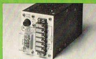
Ny strømforsyning fra Advance. Målene er 164 × 70 × 88 mm.
