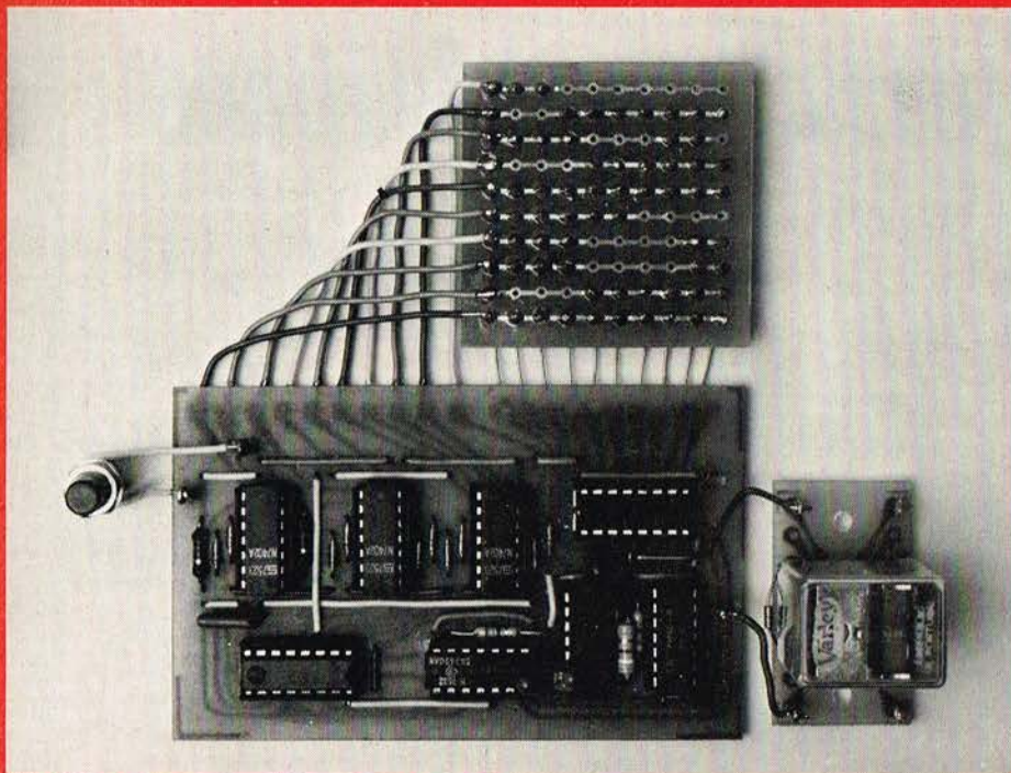
COMPACT MATRIX monteret på print og forbundet til AUTOFON.
