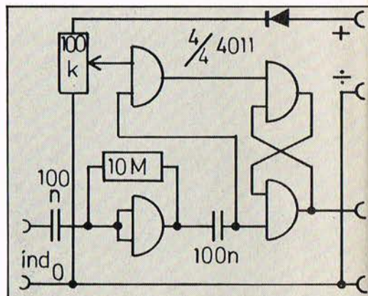
Diagram over tælleforsats.
