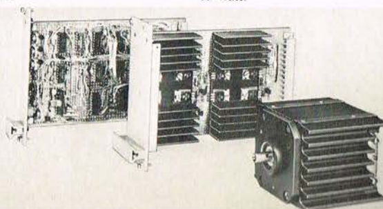
PABST motoren med den tilhørende elektronik. — Motordimensionerne er 86×90×68 mm. I fri luft er effekten 30 watt.
