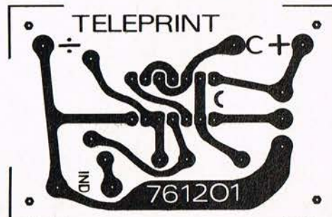
Trykt kredsløb TELEPRINT 761201 i forholdet 1:1.
