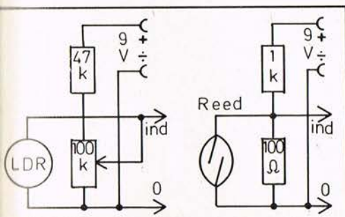
▲ Forbindelse hvis reedkontakt anvendes. Tilslutning af fotomodstand.
