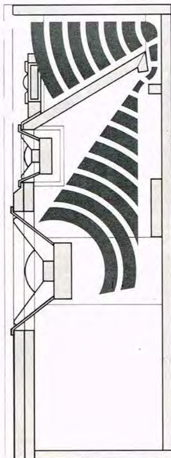
ATL højttaleren hvor basrefleksken ledes om bag diskantenhederne.
