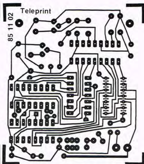
Printet set fra kobbersiden i forhold 1:1
