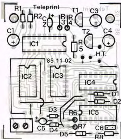
Komponentplacering.
