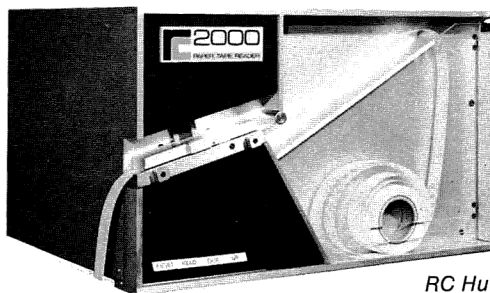
RC Hulstrimmellæsere
