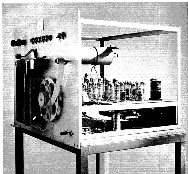
Dask læser
