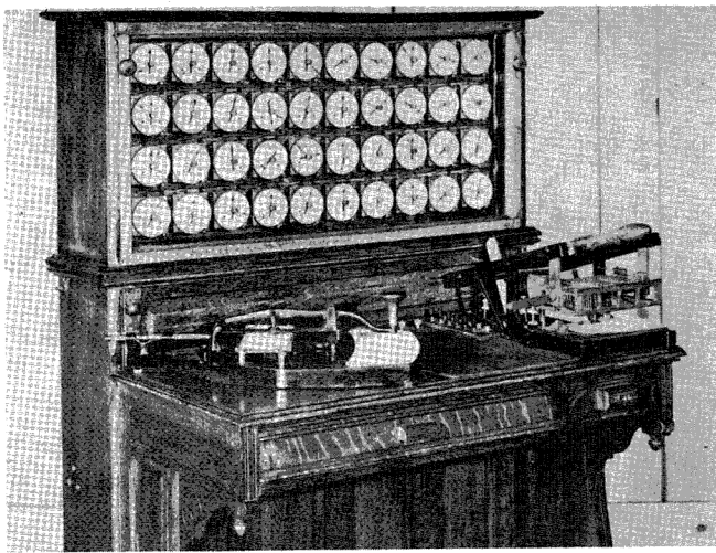
Hollerith's tabulator
