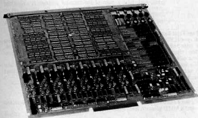
16K Memory Module 1.2 \mu s
